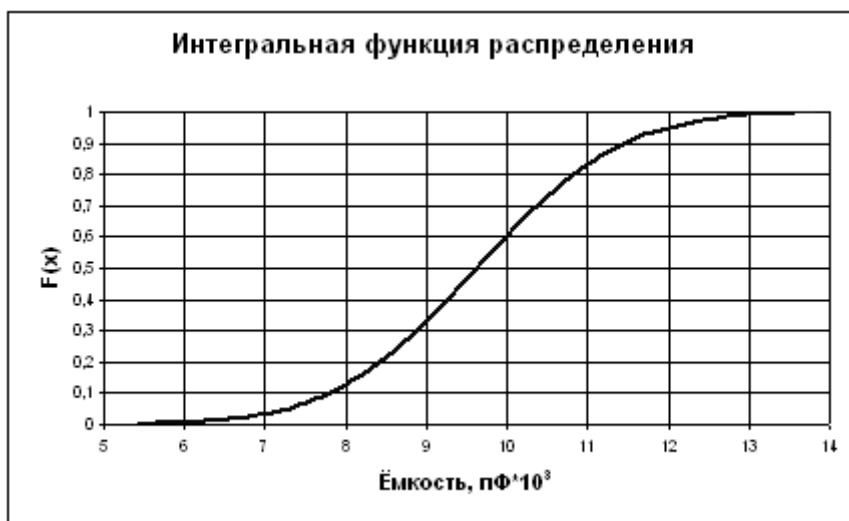
Рис. 1.2. Интегральная функция распределения ёмкости пластин пьезоэлементов Для построения графика дифференциальной функции распределения выполняем аналогичные действия. При этом на втором шаге в качестве диапазона данных выделяем диапазоны ячеек С6:С90 и Е6:Е90. Поскольку эти диапазоны находятся не в соседних столбцах, их выделение может быть сделано при нажатой клавише Ctrl. График дифференциальной функции распределения показан на рис. 1.3.
