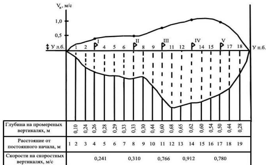
Рис. 3. Схема водного сечения (р. Уршак, с. Королёва) с эпюрой средних скоростей на вертикалях
