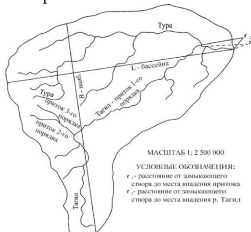
Рис. 1. Фрагмент (верхняя часть) бассейна р. Тура
