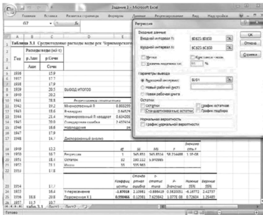
Рис. 4.1. Пример проведения регрессионного анализа в Excel
