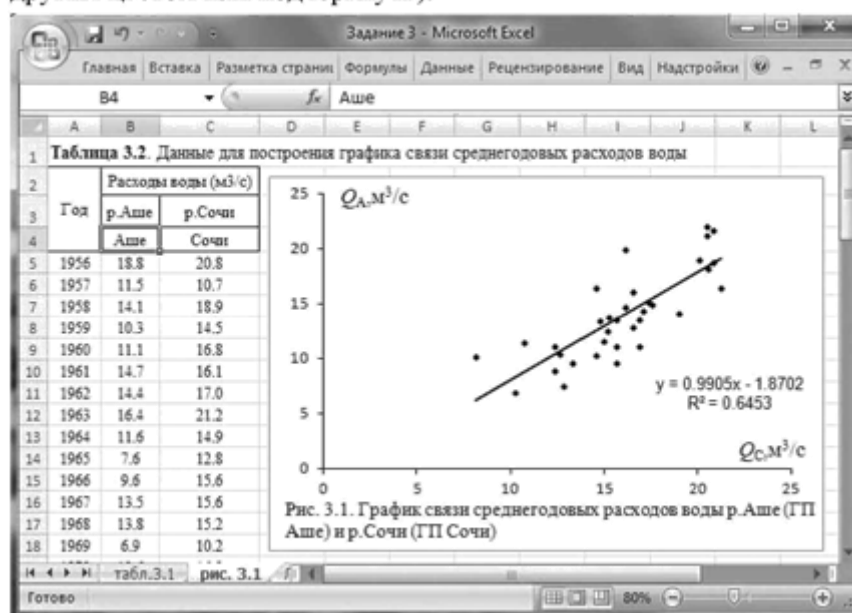
Рис. 4.2. Пример графика связи двух переменных, построенного в Excel
