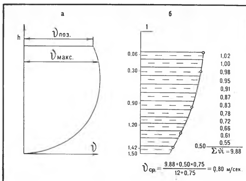
Рис. 7. Эюра скоростей (а); вычисление средней скорости по вертикали графоаналитическим способом
