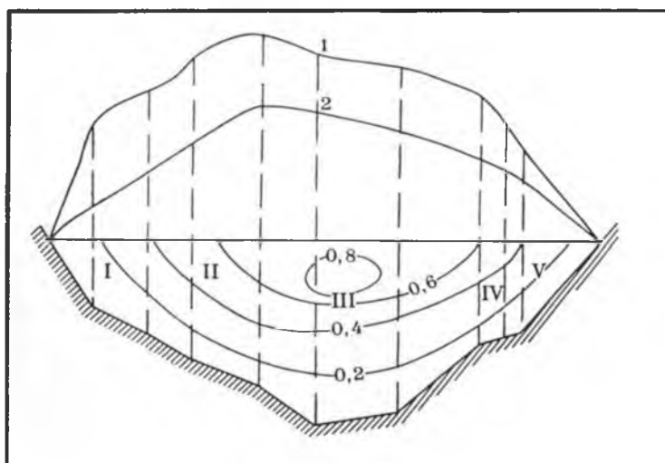
Рис. 8. Изотахи в живом сечении речного потока
