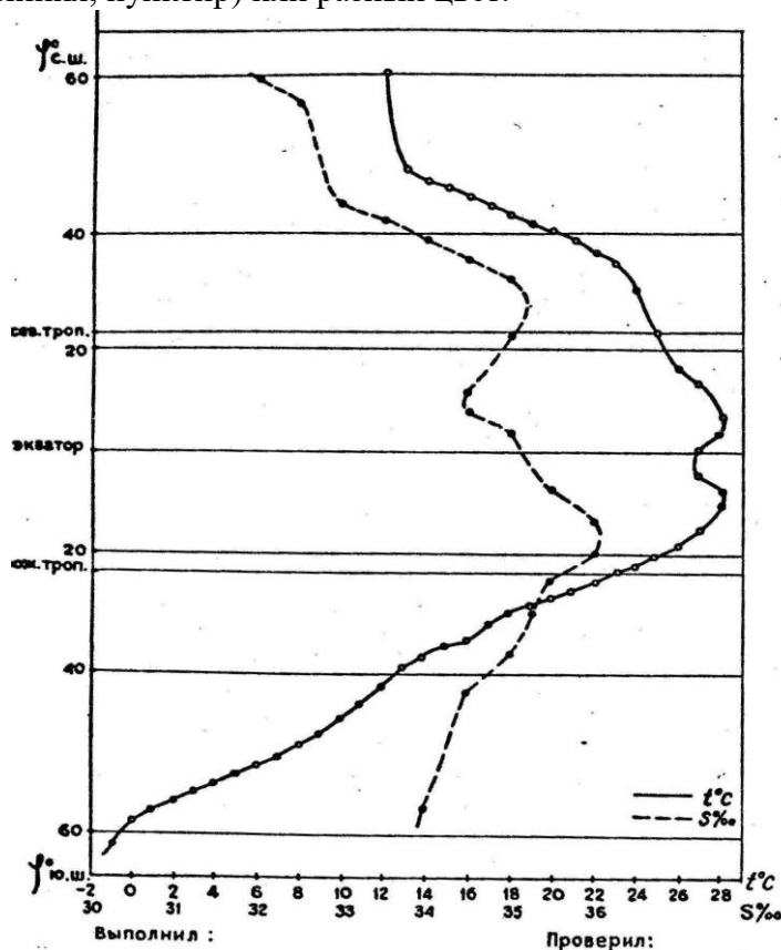
Рис. 1. Распределение температуры (t, °C) и солености (S, ‰) воды на поверхности Тихого океана в августе по меридиану 150° з.д. (пример)
