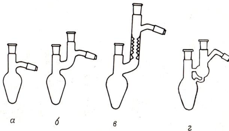
Рис. 2. Перегонка при пониженном давлении Перегонные колбы: а - грушевидная; б - Кляйзена; в - Кляйзена с насадкой Вюргца; г - Арбузова.
