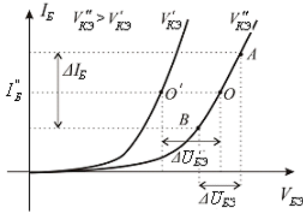
Рис.3.2. К определению h_{11\varnothing} и h_{12\varnothing} параметров биполярного транзистора.
