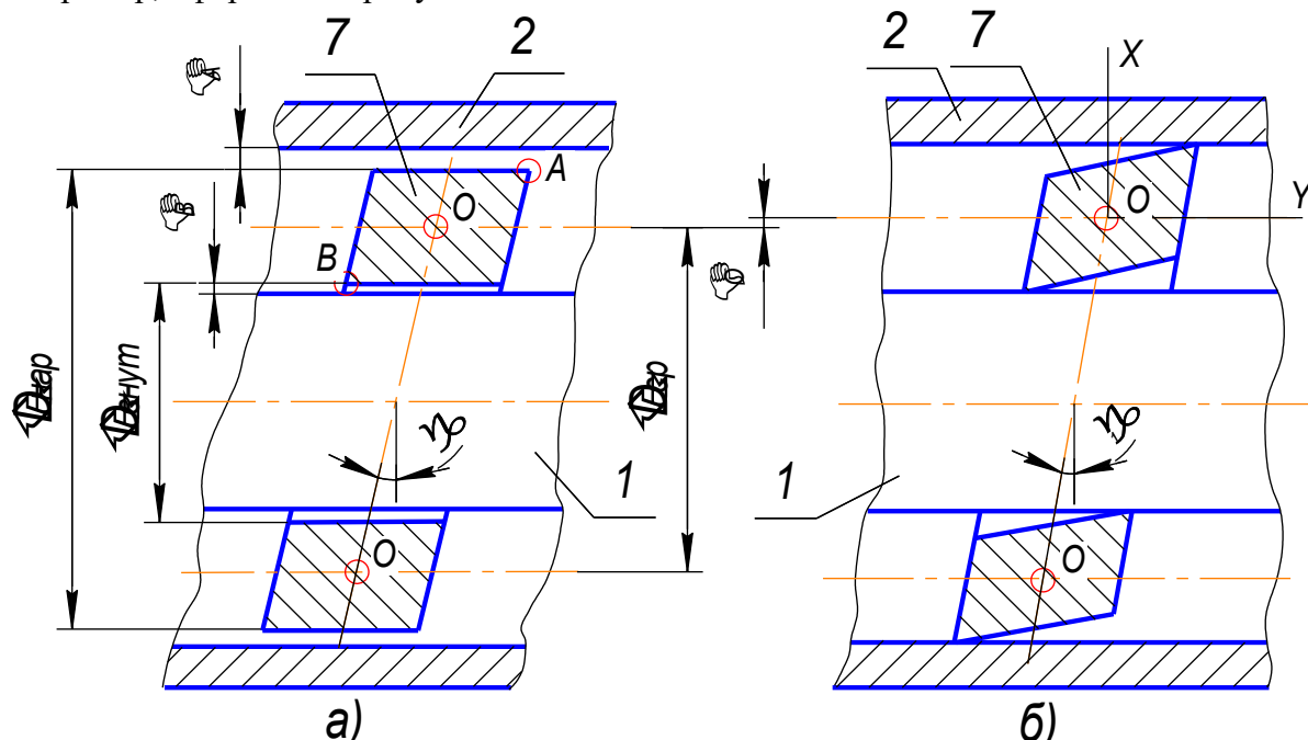
2 – приводной шпindelь, 7 – центрирующий элемент (пружина)
