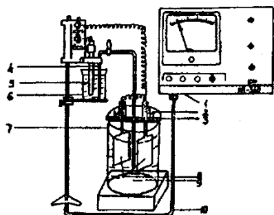
1 - милливольтметр; 2 - контактная клемма; 3 - изолирующая пластина; 4 - электролитический мостик; 5 - хлорсеребряный электрод сравнения; 6 - раствор KCl , 7 - стеклянный стакан; 8 - рабочие электроды; 9 - рабочий раствор; 10 - коаксиальный кабель
