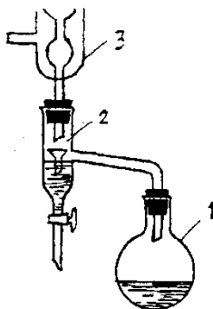
Прибор для удаления воды из реакционной смеси: 1 - колба; 2 - ловушка; 3 - холодильник
