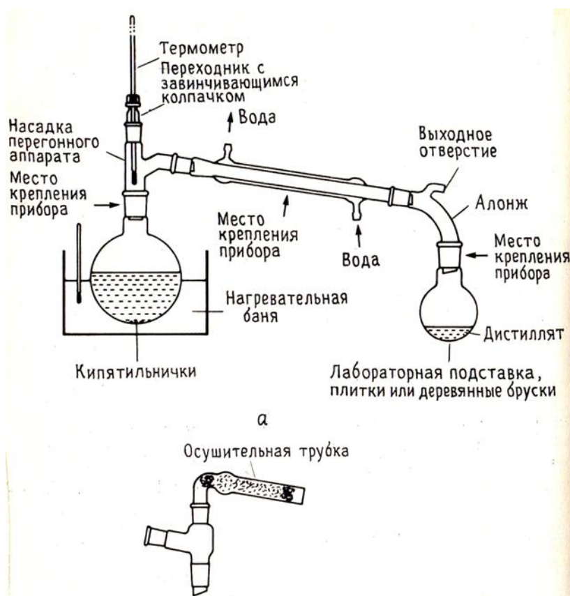
Рис.1. Простая перегонка
