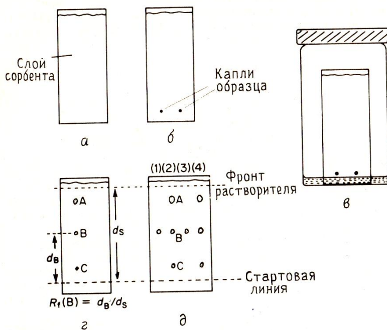
Рис.8. Тонкослойная хроматография.
