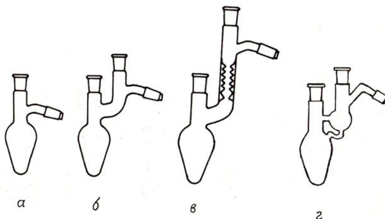
Рис. 2. Перегонка при пониженном давлении Перегонные колбы: а - грушевидная; б - Кляйзена; в - Кляйзена с насадкой Вюрге; г - Арбузова.
