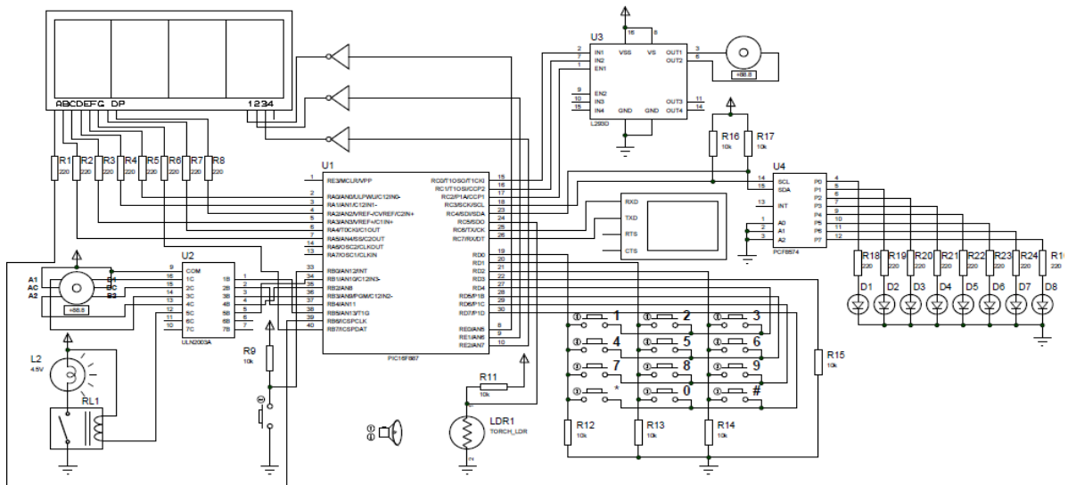
Рис. 1. Модель станда № 2 в среде моделирования Proteus ISIS Professional
