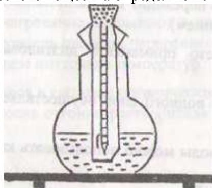
Рис.5. а – сублимация микроколичеств с использованием нагревательного блока, б – трубка для перегонки микроколичеств.
