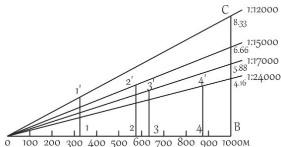
Рис. 4. Клиновый масштаб
