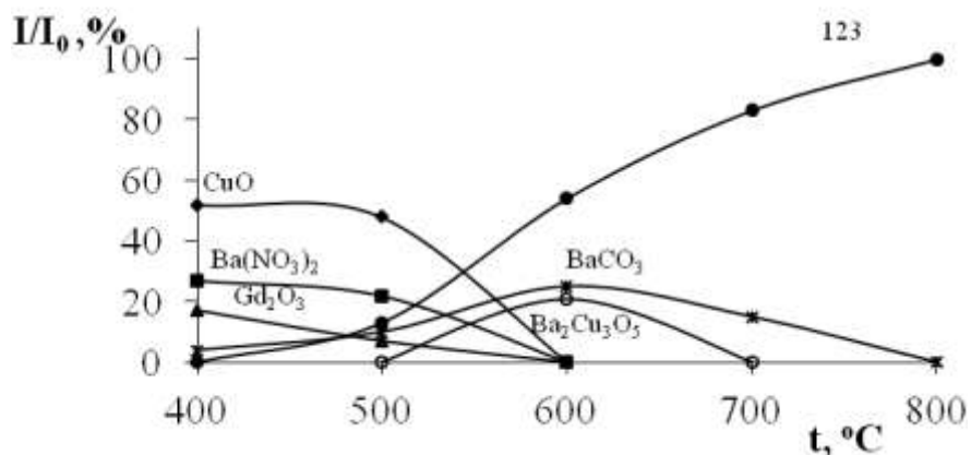
Рис.1. Последовательность фазовых превращений соединения \text{GdBa}_2\text{Cu}_3(\text{NO}_3)_{13} \cdot 9\text{C}_5\text{H}_5\text{N} \cdot \text{HNO}_3 \cdot n\text{H}_2\text{O}
