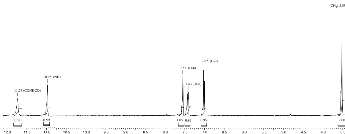
Рисунок 2.23. Спектр ЯМР ^1\text{H} 7-бром-1,5-дигидро-2Н-хромено-[2,3-d]пиримидин-2,4(3Н)-диона
