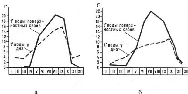
Рис. 7. Внутригодовой ход средних месячных температур воды озер: а - Чебаркуль, б - Тургояк
