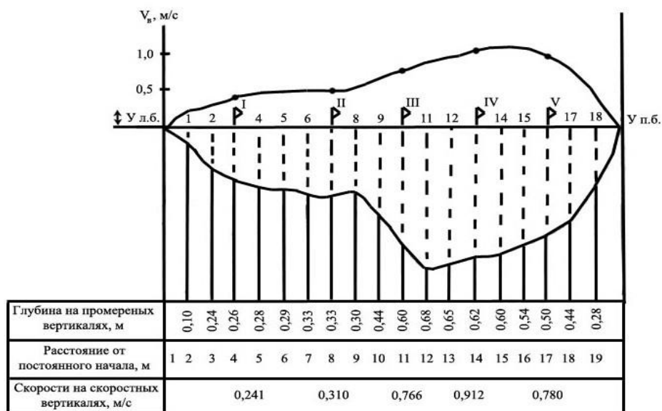
Рис. 3. Схема водного сечения (р. Уршак, с. Королёва) с эпорой средних скоростей на вертикалях
