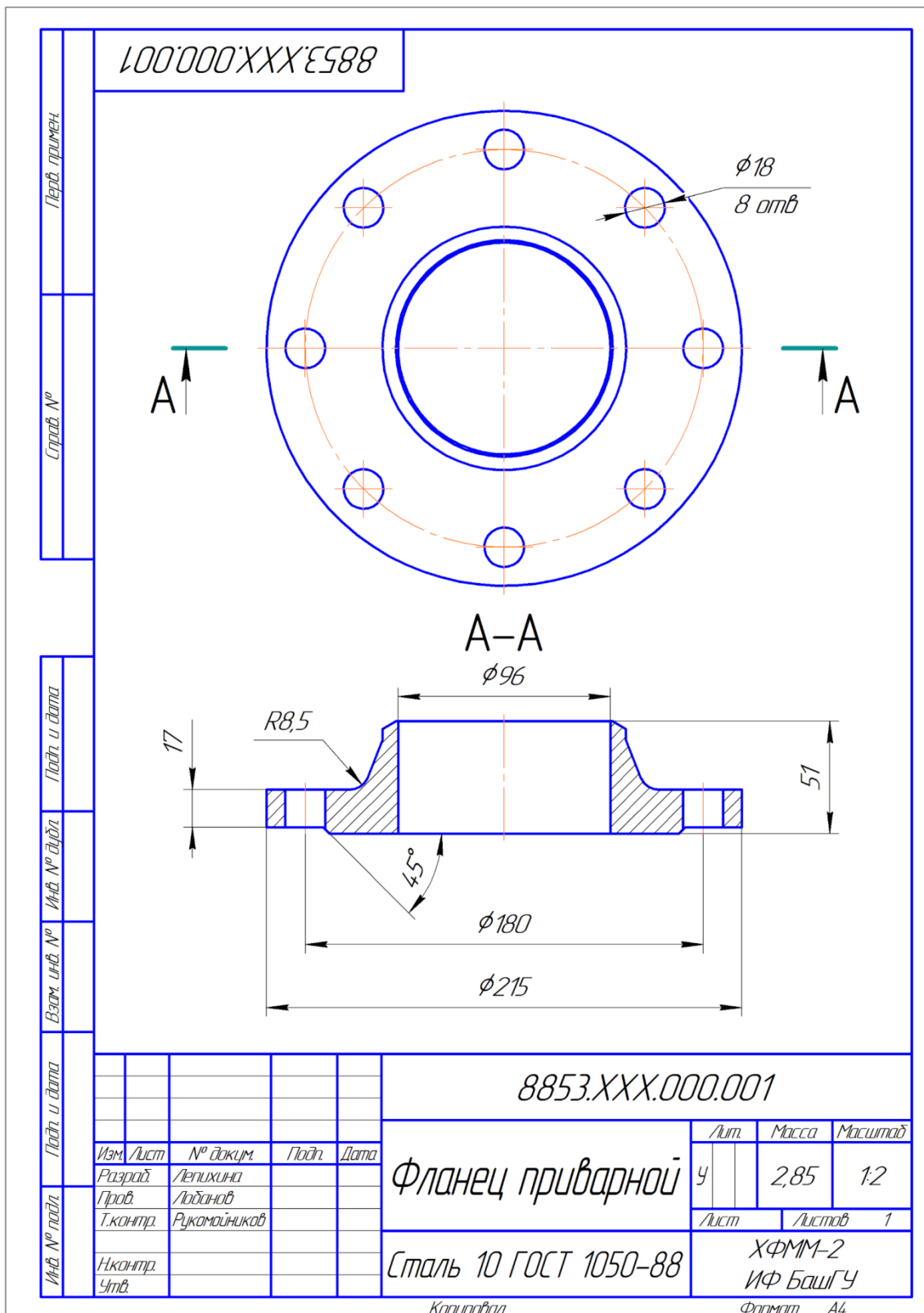
Рисунок 1.3 - Чертеж детали
