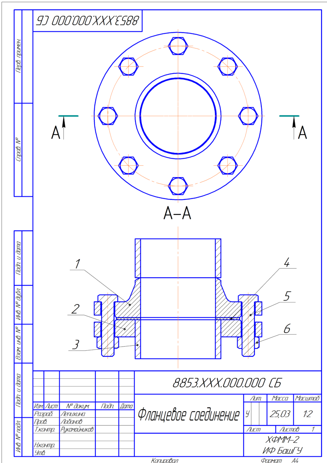
Рисунок 1.2 - Сборочный чертеж
