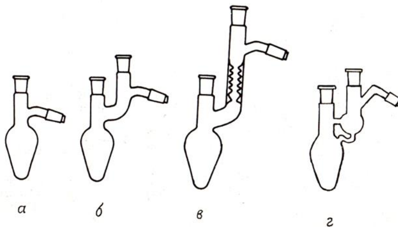
Рис. 2. Перегонка при пониженном давлении Перегонные колбы: а - грушевидная; б - Кляйзена; в - Кляйзена с насадкой Вюрца; г - Арбузова.
