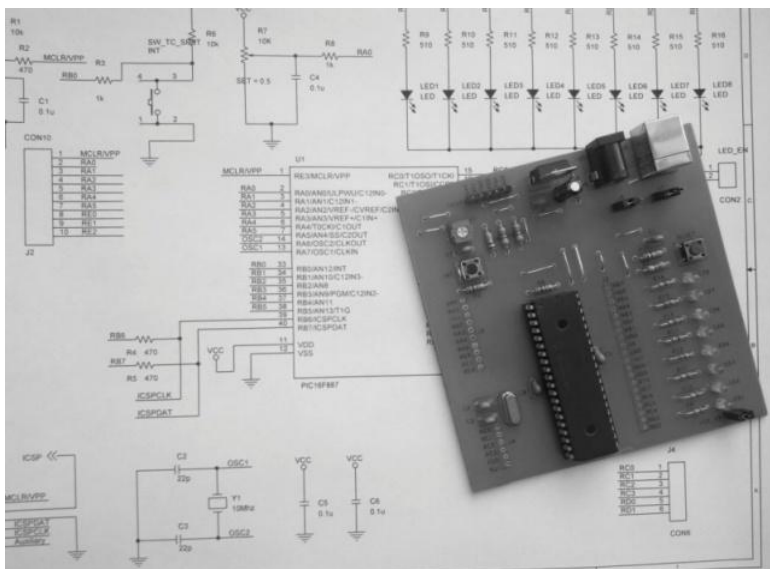
Рис. 3. Лабораторный стенд № 3
