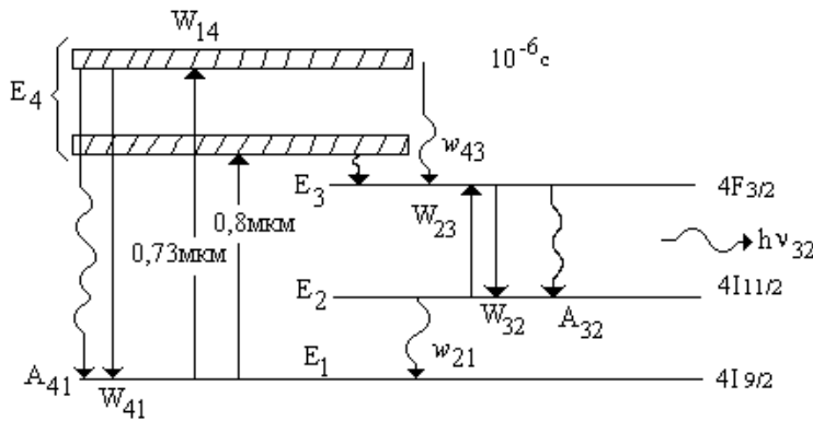
Рис.1. Схема энергетических уровней Nd^{3+} в кристалле граната.
