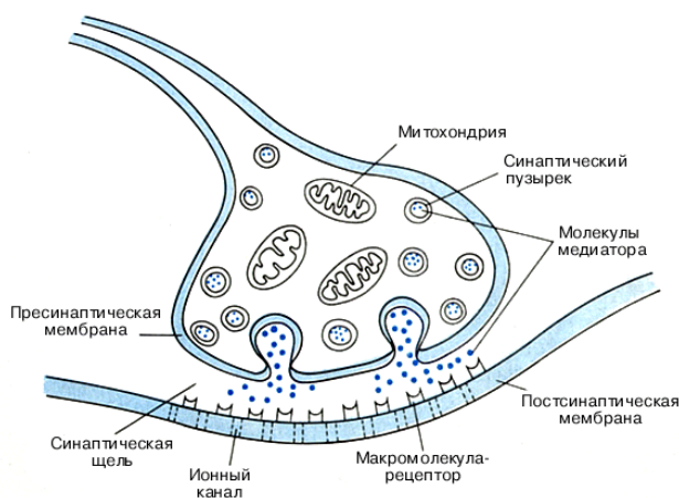
Рис1. Строение синапса.
