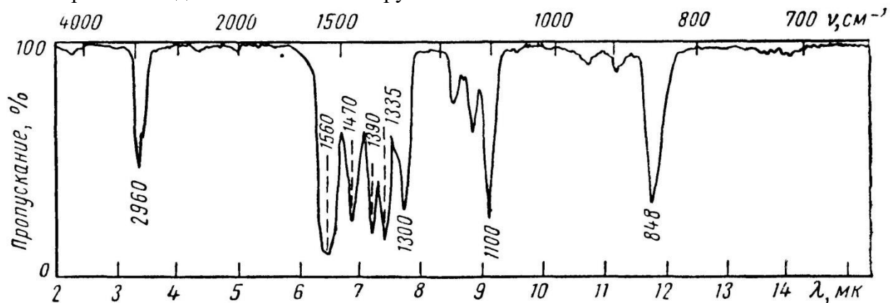
Рис 1. \text{C}_8\text{H}_8\text{O}_2
