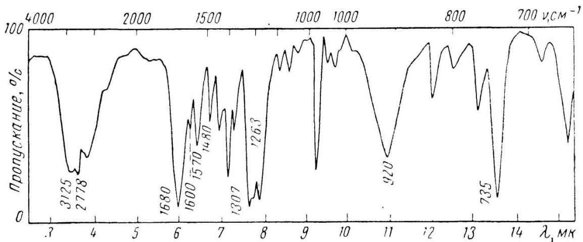
Рис 2. \text{C}_7\text{H}_{13}\text{ON}
