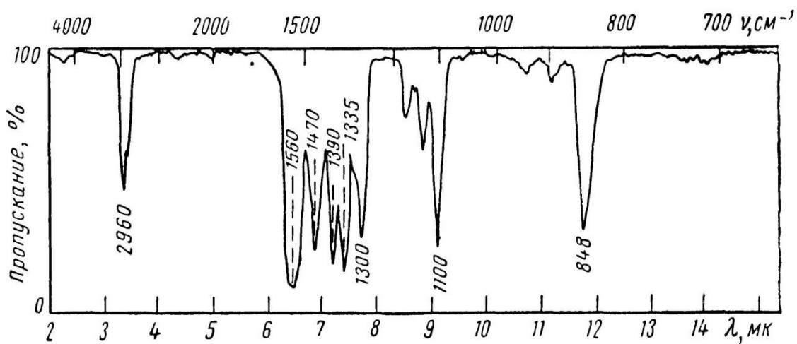
Рис 3. \text{C}_3\text{H}_7\text{O}_2
