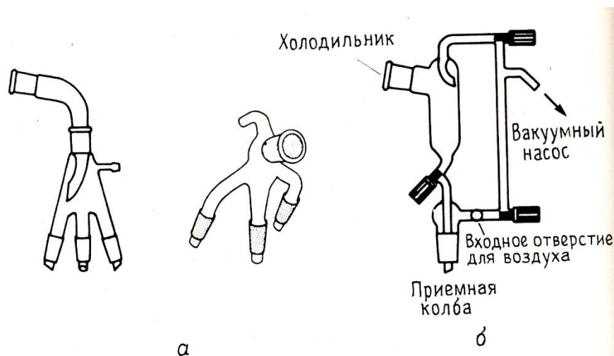
Рис.3 Типы алонжей: а – вращаемый многолапчатый «паук», б – форштос Перкина.
