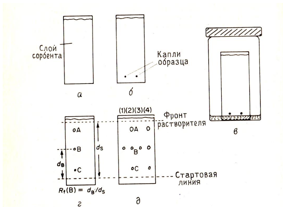
Рис.8. Тонкослойная хроматография.
