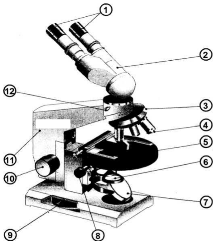
Рис. 1. Микроскоп с бинокулярной насадкой и зеркалом: I - окуляры; 2 - бинокулярная насадка; 3 - «револьвер»; 4 - объектив; 5 — предметный столик; 6—конденсор; 7—зеркало; 8 —рукоятка перемещениякронштейна конденсора; 9 -рукоятка тонкой фокусировки (микровинт); 10 — рукоятка грубой фокусировки (макровинт); II- тубусодержатель; 12 - винт для крепления бинокулярной насадки
