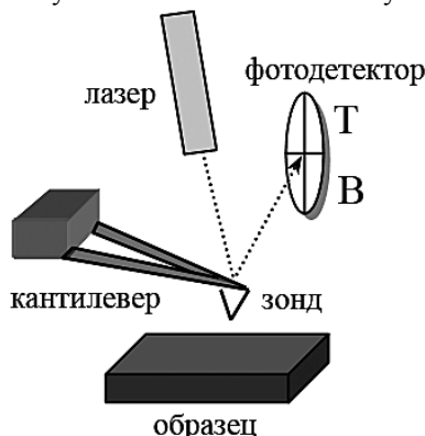
Рис.1 Схема силового датчика
