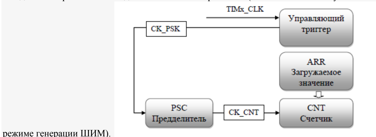
Рис. 2.1. Схема управления подсчетом импульсов
