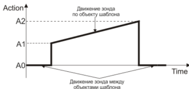
Рис. 2. Процесс проведения градиентной литографии
