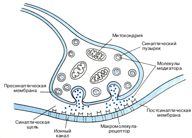
Рис1. Строение синапса.
