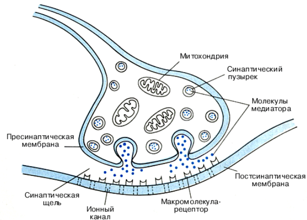
Рис1. Строение синапса.
