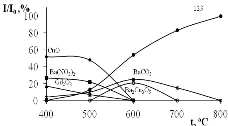
Рис.1. Последовательность фазовых превращений соединения \text{GdBa}_2\text{Cu}_3(\text{NO}_3)_{13} \cdot 9\text{C}_2\text{H}_5\text{N} \cdot \text{HNO}_3 \cdot n\text{H}_2\text{O}
