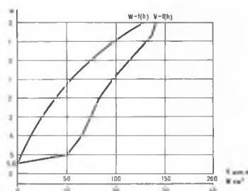
Рис. 4. Кривые площадей и объемов озера Смолино
