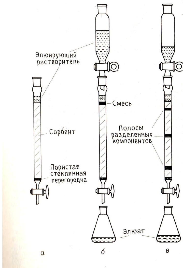
Рис.9. Колоночная хроматография (с «гравитационным» элюированием т. е. под действием собственной силы тяжести)
