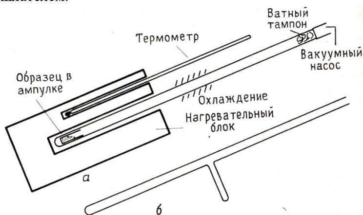
Рис.5. а – сублимация микроколичеств с использованием нагревательного блока, б – трубка для перегонки микроколичеств.
