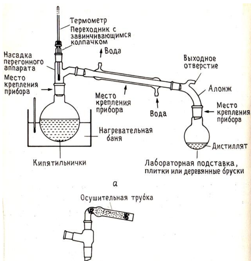
Рис.1. Простая перегонка
