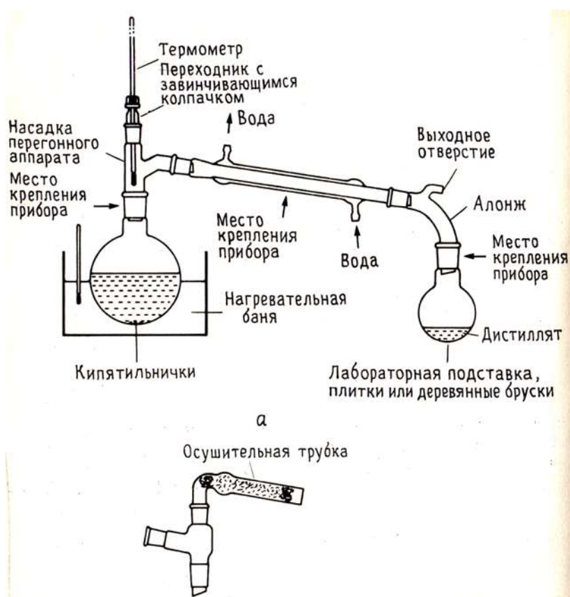
Рис.1. Простая перегонка
