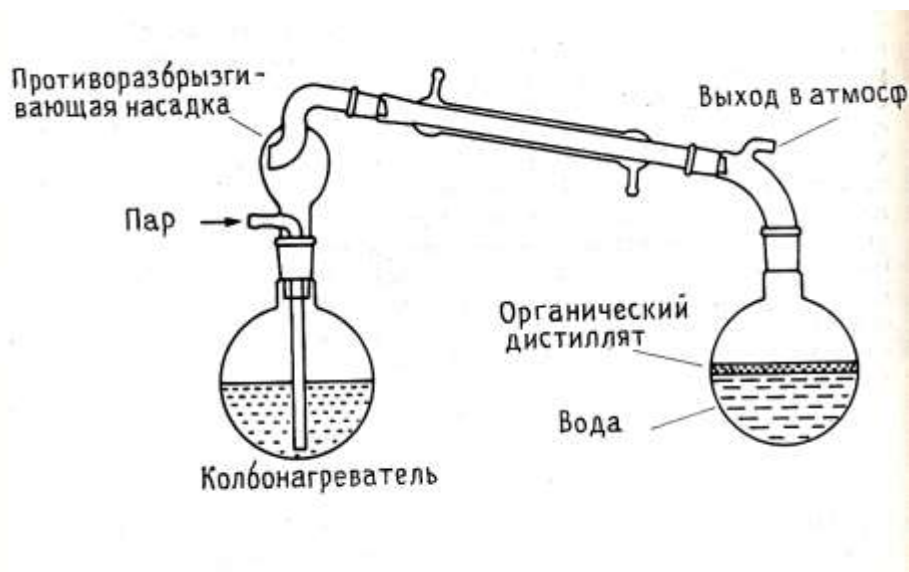
Рис.4 Прибор для перегонки с водяным паром.
