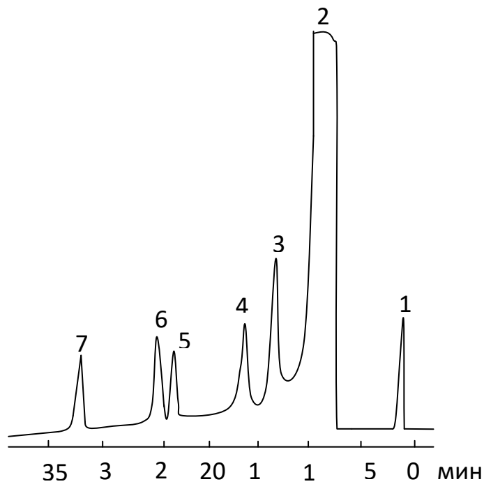
Рис. 2. Хроматограмма
