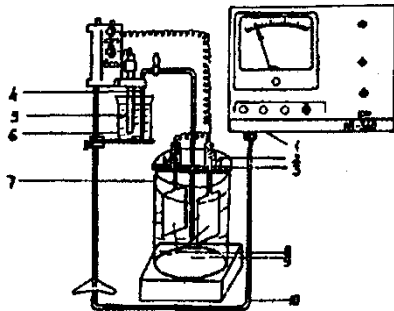
1 - милливольтметр; 2 - контактная клемма; 3 - изолирующая пластина; 4 - электролитический мостик; 5 - хлорсе-ребрянный электрод сравнения; 6 - раствор KCl , 7 - стеклянный стакан; 8 - рабочие электроды; 9 - рабочий раствор; 10 - коаксиальный кабель
