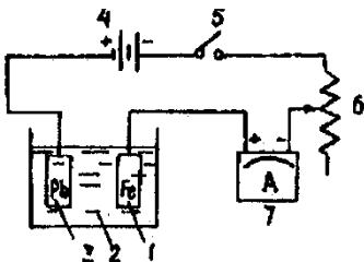
1 - защищаемый образец; 2 - агрессивный раствор; 3 - вспомогательный электрод; 4 - источник тока (выпрямитель); 5 - ключ; 6 - реостат; 7 - амперметр
