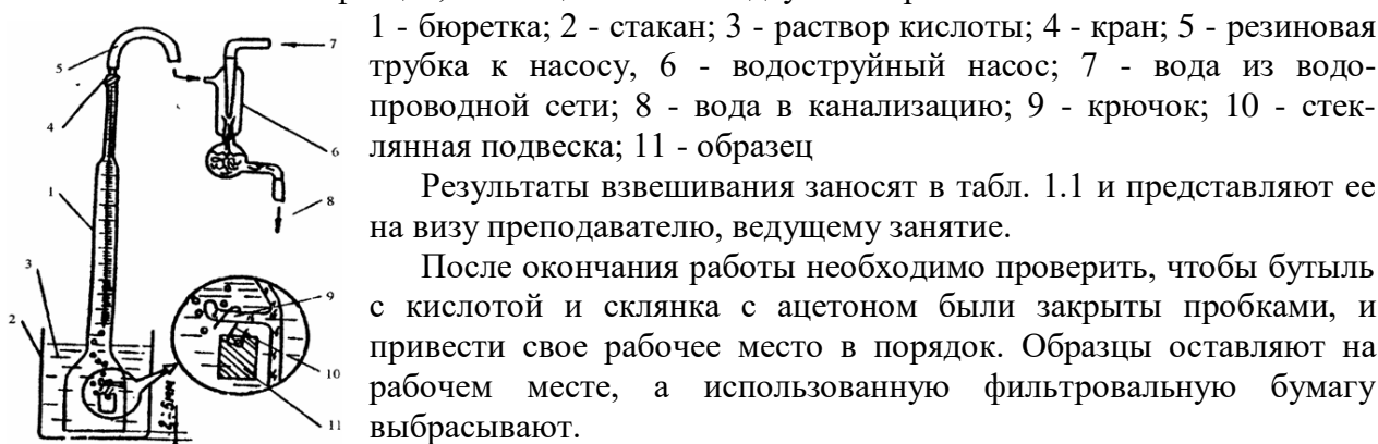
Рис. 1. Схема установки для изучения кинетики
