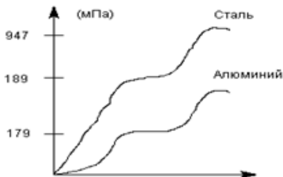
Рисунок 1.2 - Диаграмма растяжения стального и алюминиевого образцов
