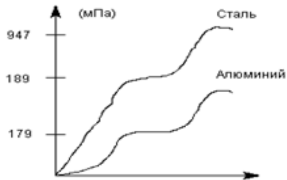
Рисунок 1.2 - Диаграмма растяжения стального и алюминиевого образцов
